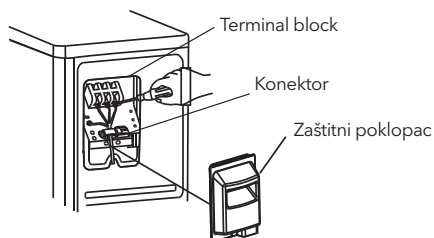
Shema konekcije
