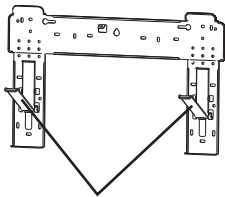
Shpalosni kllapa në pllakën e montimit
