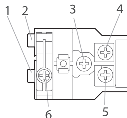
priključna kutija
