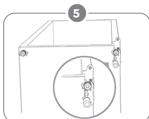
Odvrtite donju šarku. Zatim uklonite podvesne nožice sa obe strane.
