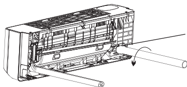
Σφίξτε (αντίστροφα) το σωλήνα φρέσκου αέρα
