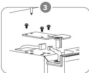
Odšarafite gornju šarku.
