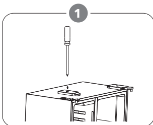
Odšarafite polopac šarke Filipsovim odvrtlačem.
