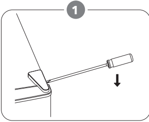
1 Odstranite pokrov zgornjega desnega tečaja.
