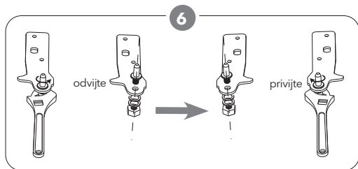
6 S ploškim izvijačem odvijte spodnji zatič tečaja in ga odstranite, nato pa obrnite nosilec in zamenjajte zatič.
