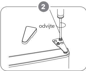
2 Odstranite vijake. Nato odstranite nosilec tečaja.
